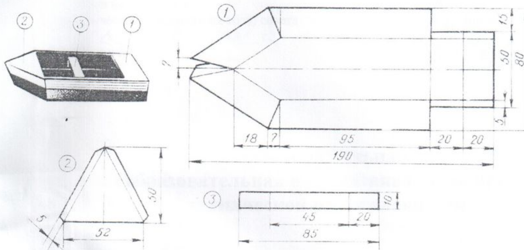
Рис. 1. Модель лодки-плоскодонки: 1 – корпус лодки; 2 – носовая часть; 3 – банка.
